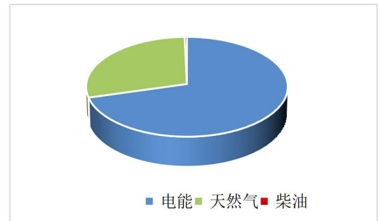
2022年能源结构分布图
