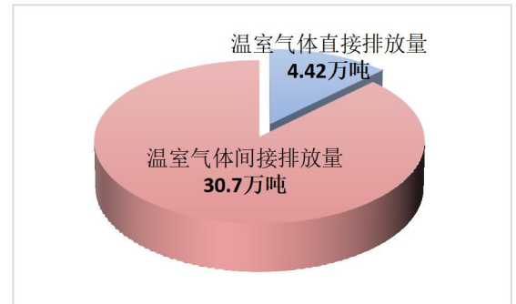
2022年温室气体（CO 2 ）排放情况
